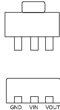
SOT-89
